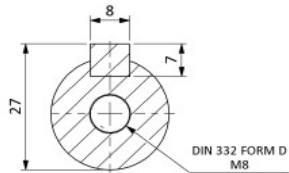
KESİT A-A
